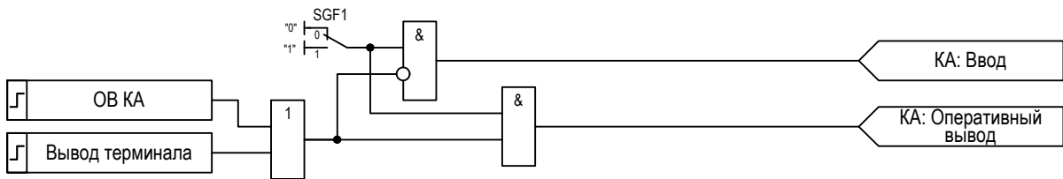
Рисунок 2.32 – Логика управления режимами функционального блока «КА»
